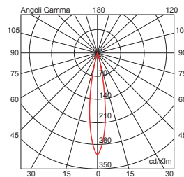
Emissione a fascio stretto/medio/largo / Spot/Medium/Diffuse beam
