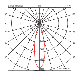
Emissione a fascio stretto/medio/largo / Spot/Medium/Diffuse beam
