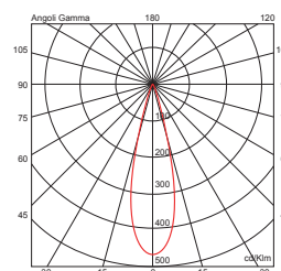
Emissione a fascio stretto/medio/largo / Spot/Medium/Diffuse beam
