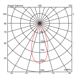
Emissione a fascio stretto/medio/largo / Spot/Medium/Diffuse beam
