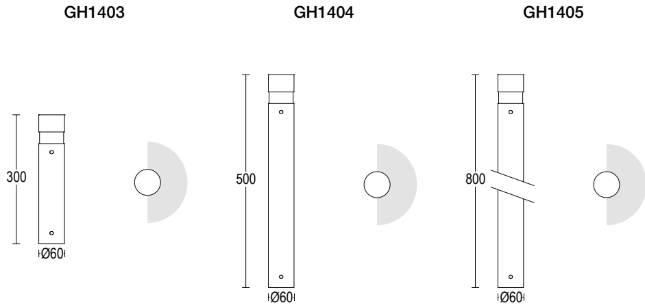
MiniTondo Dark 300 180° MiniTondo Dark 500 180° MiniTondo Dark 800 180°
